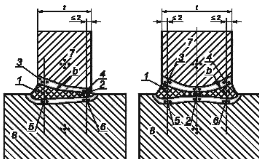
д) Расположение отпечатков при толщине основного металла и глубине сварного шва h или t не менее 4 мм
