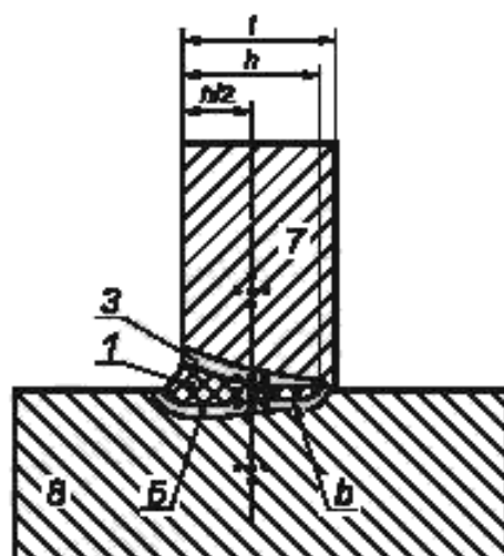
с) Расположение отпечатков при толщине основного металла и глубине сварного шва h или t не более 4 мм
