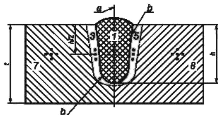
а) Расположение отпечатков при глубине сварного шва h менее 4 мм
