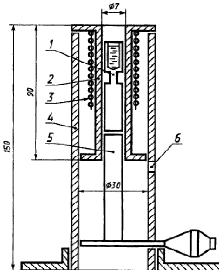
1 — электрод с пробой; 2 — кварцевая трубка; 3 — нагреватель на 300 Вт; 4 — корпус печи; 5 — толкатель; 6 — фиксатор
